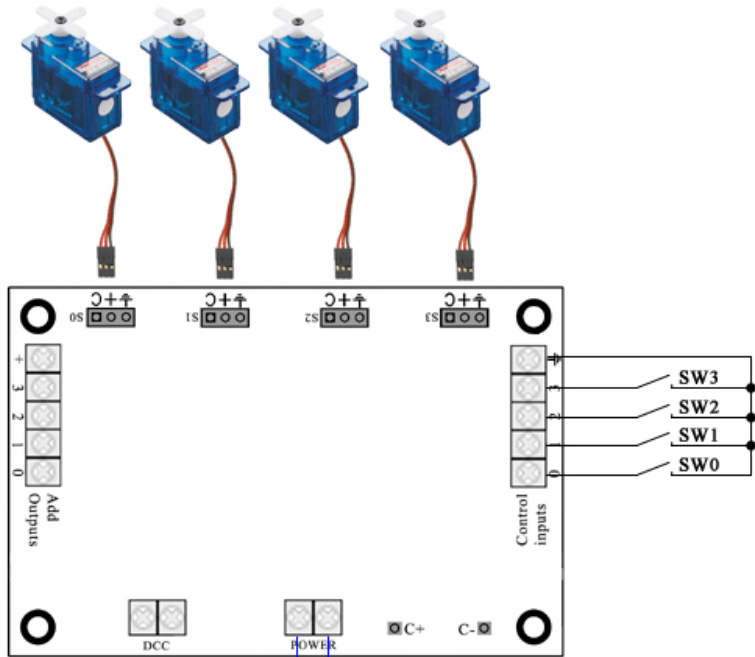
К источнику питания Ручное управление стрелками
