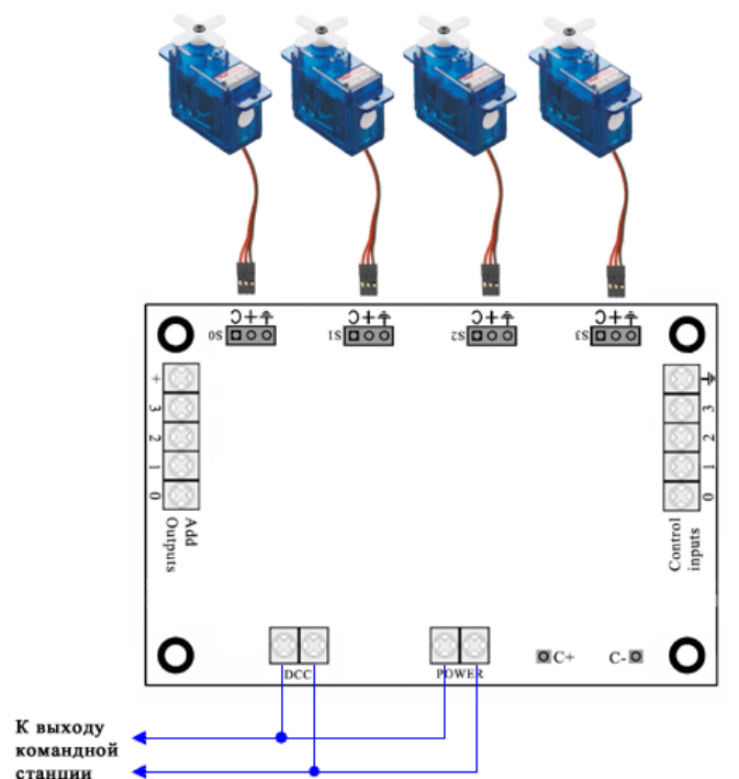
Схема простого включения. Питание берется с рельс
